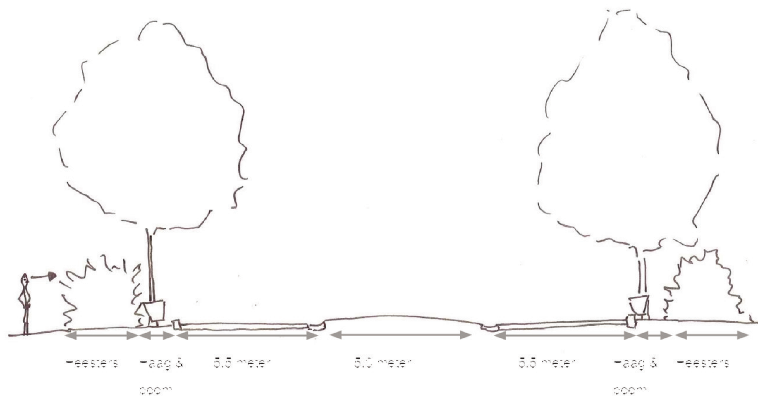
Afbeelding 42. Doorsnede van een nieuwe laan met een centrale beplantingsstrook. Een nieuwe structuur die de mozaïekachtige esrand versterkt. Ook vanuit ecologisch oogpunt is deze structuur aantrekkelijk.
