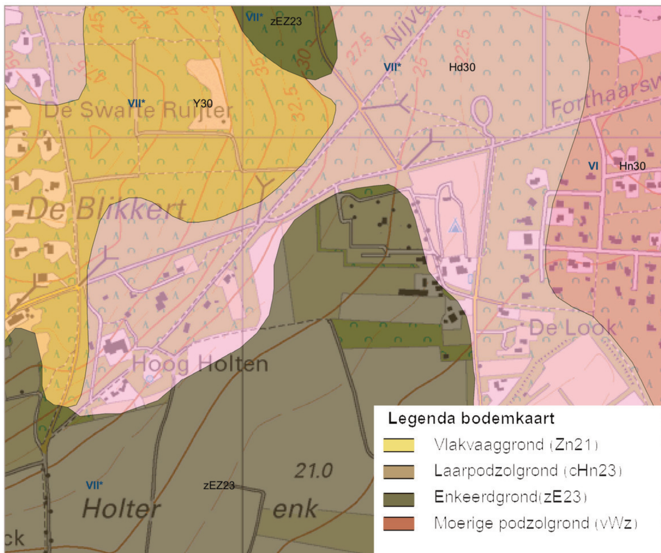
Afbeelding 9. Bodemkaart projectgebied en omgeving
