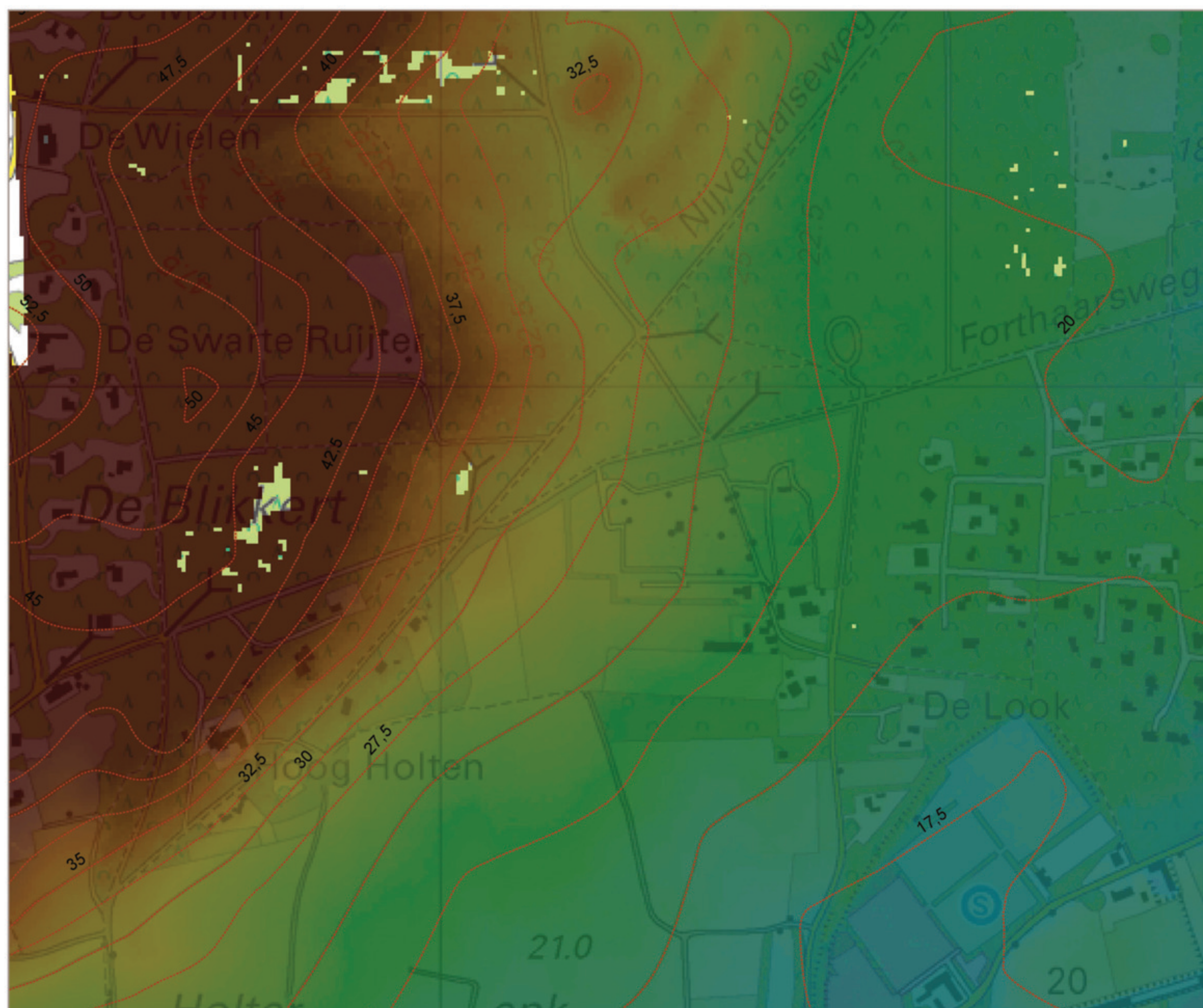
Afbeelding 10. Hoogtekaart projectgebied en omgeving
