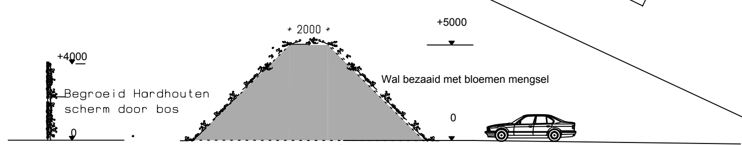
Doorsnede C
