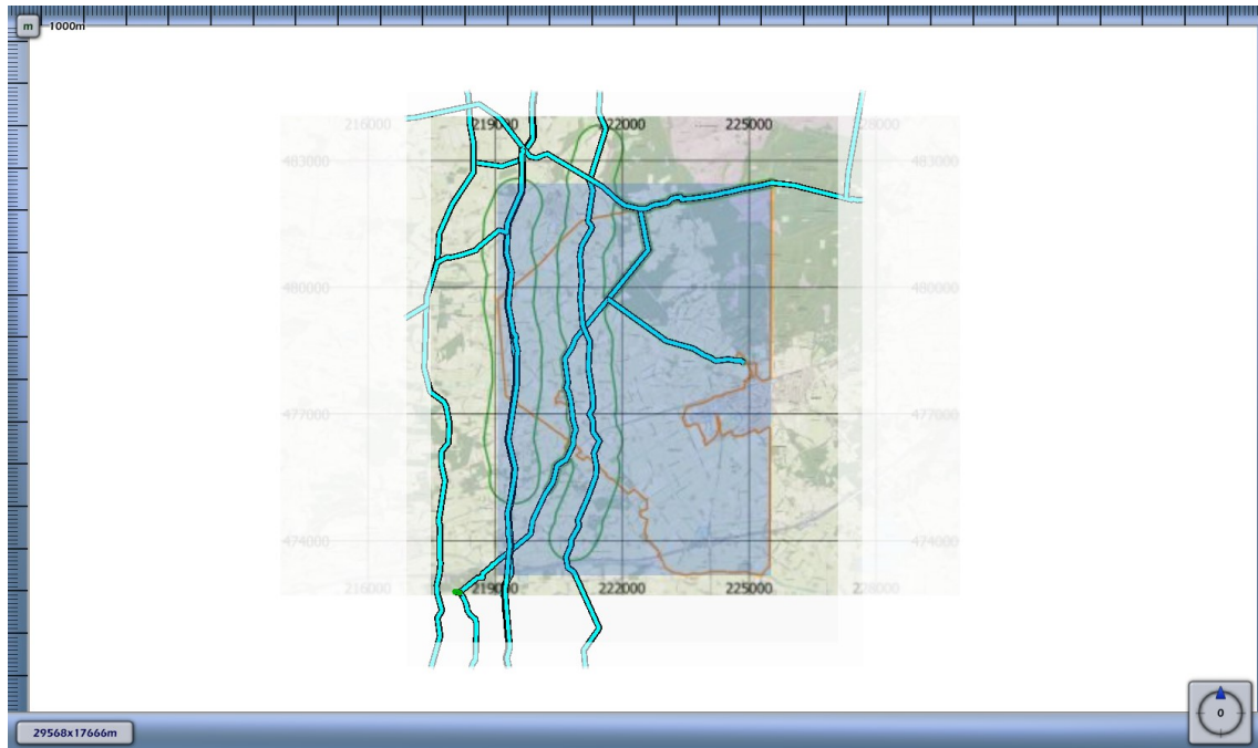
3.20 Figuur 3.20 Plaatsgebonden risico voor 4759_leiding-N-558-40-deel-1 van N.V. Nederlandse Gasunie
