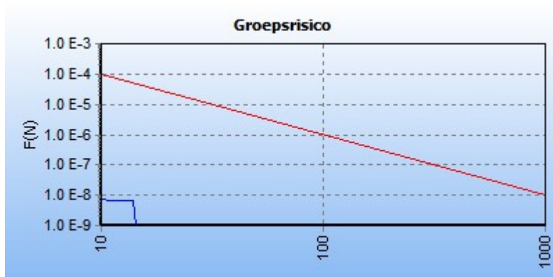
5.11 Figuur 5.11 FN curve voor 4759_leiding-A-588-deel-1 van N.V. Nederlandse Gasunie voor de kilometer tussen stationing 3710.00 en stationing 4710.00
