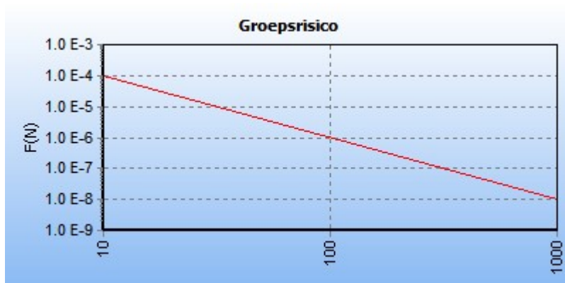
5.5 Figuur 5.5 FN curve voor 4759_leiding-A-511-deel-1 van N.V. Nederlandse Gasunie voor de kilometer tussen stationing 630.00 en stationing 1630.00
