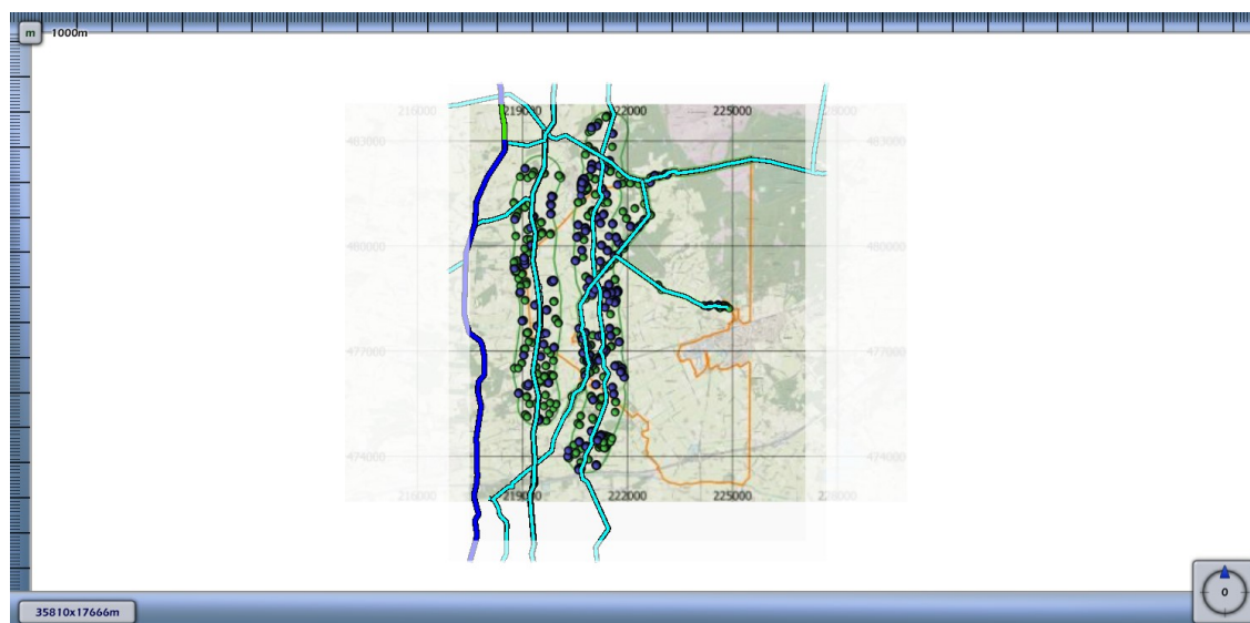
Figuur 4.5 Kilometer leiding behorende bij de maximale overschrijding van de FN-curve voor 4759_leiding-A-511-deel-1 van N.V. Nederlandse Gasunie
