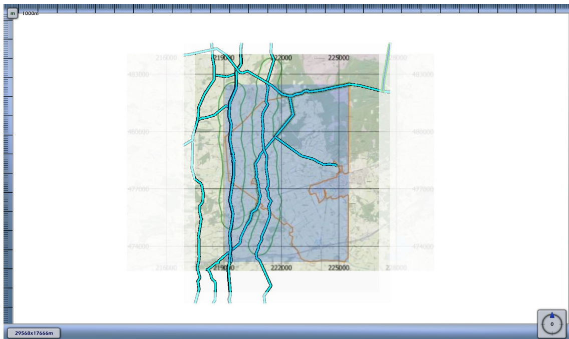
3.16 Figuur 3.16 Plaatsgebonden risico voor 4759_leiding-N-557-32-deel-1 van N.V. Nederlandse Gasunie
