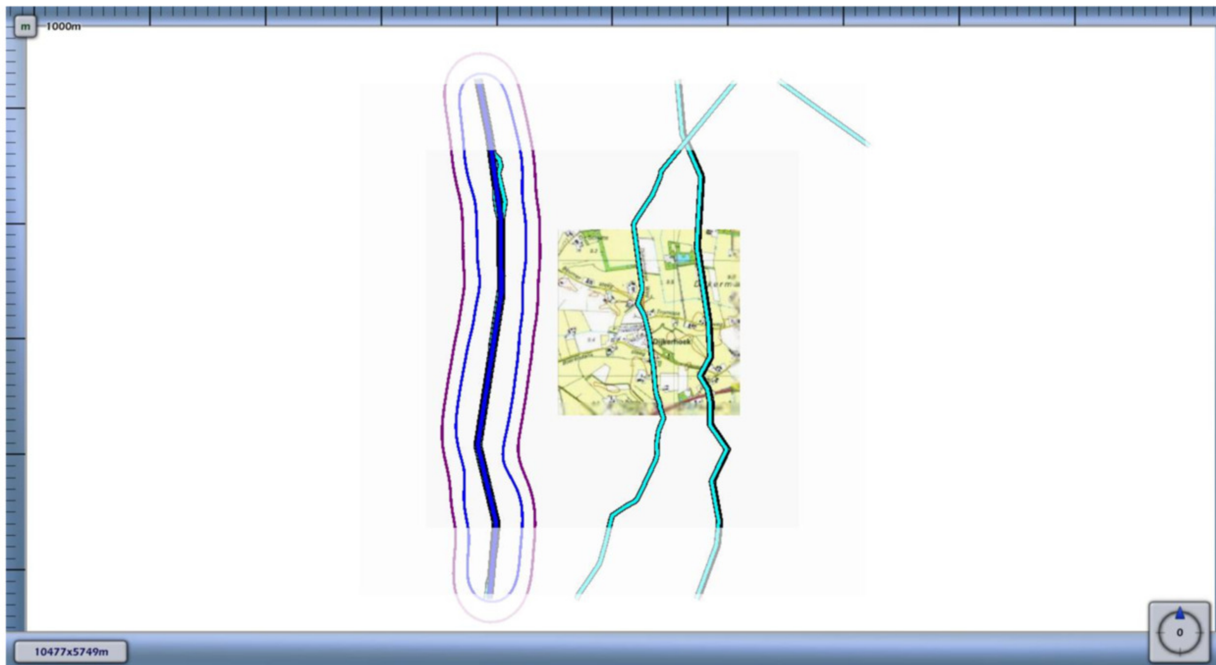
3.2 Figuur 3.2 Plaatsgebonden risico voor A-506 van N.V. Nederlandse Gasunie
