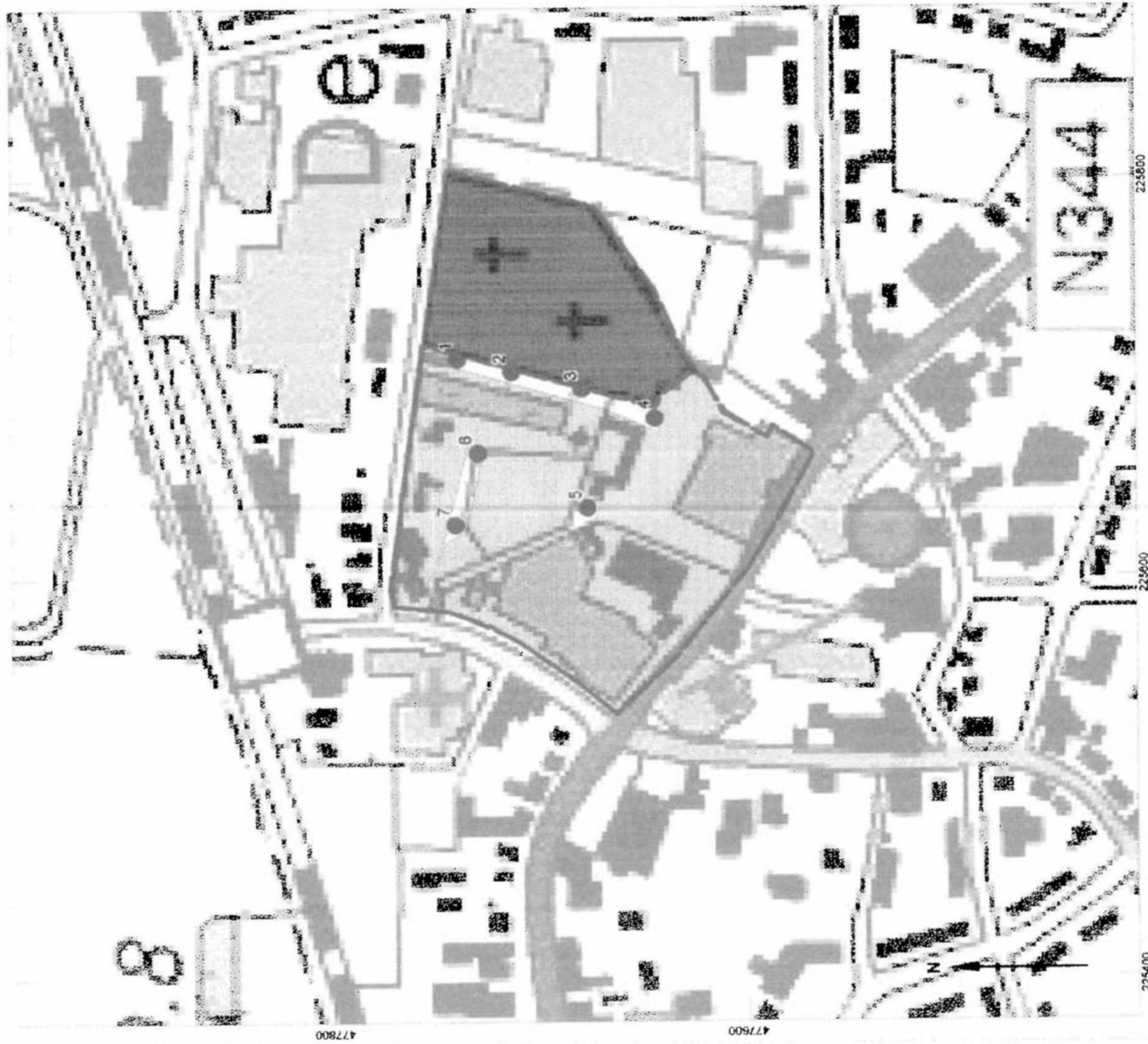
AFBEELDING 5 BOORPUNTENKAART
