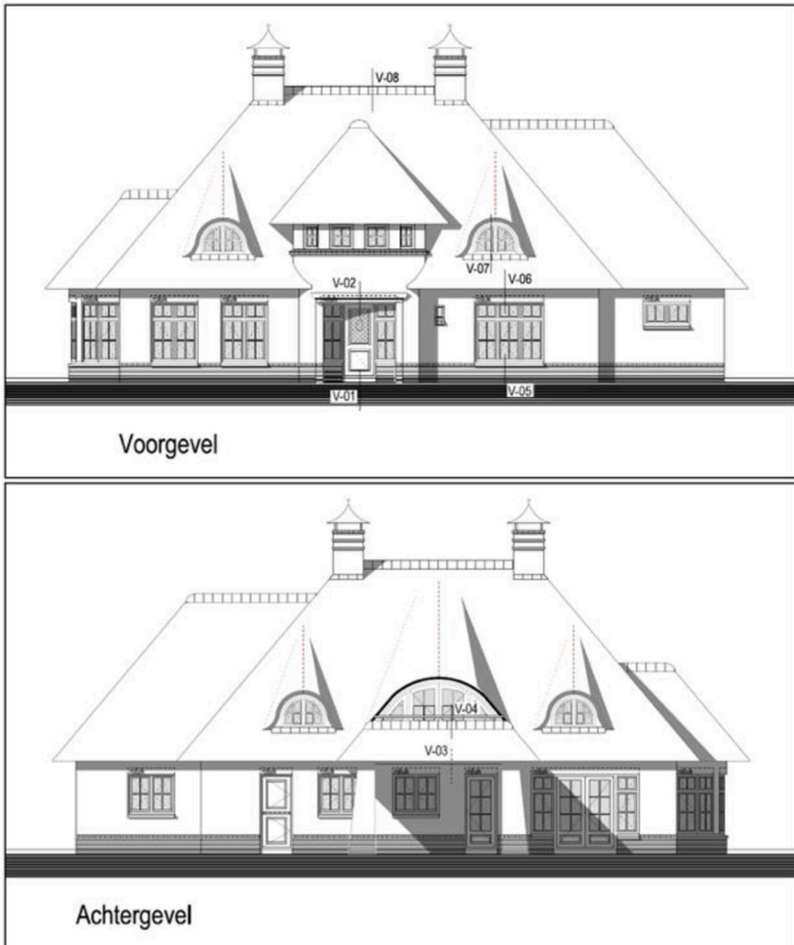
Afbeelding 2.4 Voorgevel- en achtergevelaanzicht vervangende woning (Bron: 01 Architecten)
