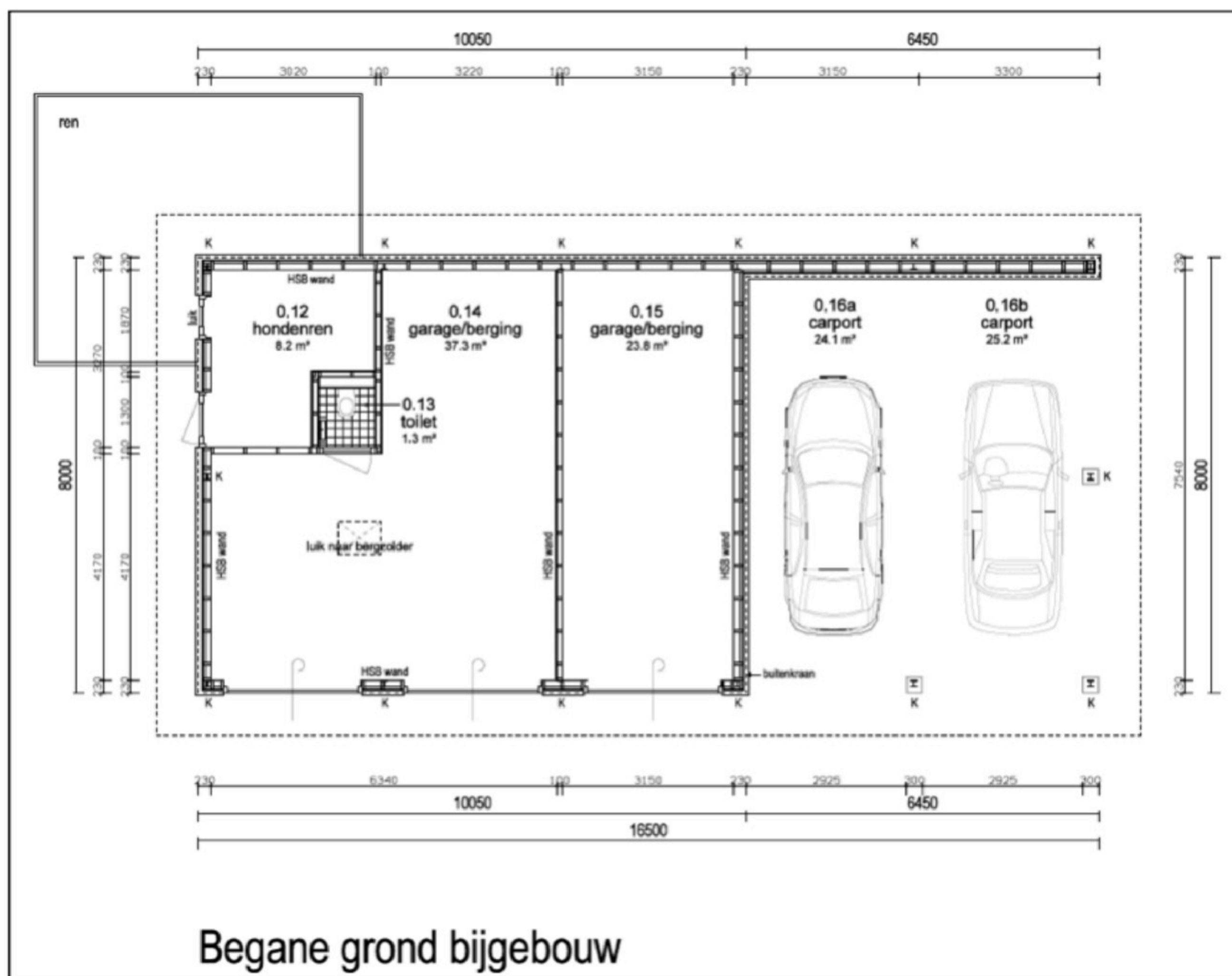
Afbeelding 2.5 Plattegrond van het nieuwe bijgebouw (Bron: 01 Architecten)
