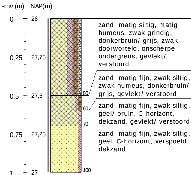
Boring 3 RD-coördinaten: 232132/479742
