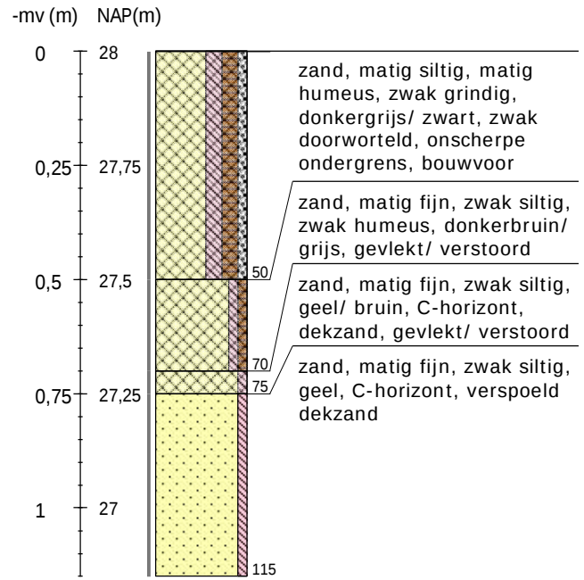
Boring 2 RD-coördinaten: 231133/479759
