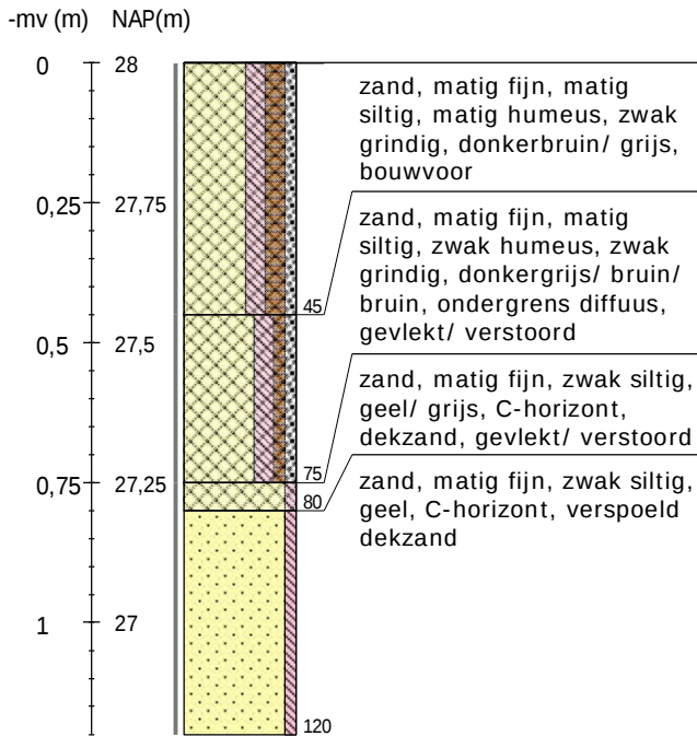
Boring 3 RD-coördinaten: 232132/479742
